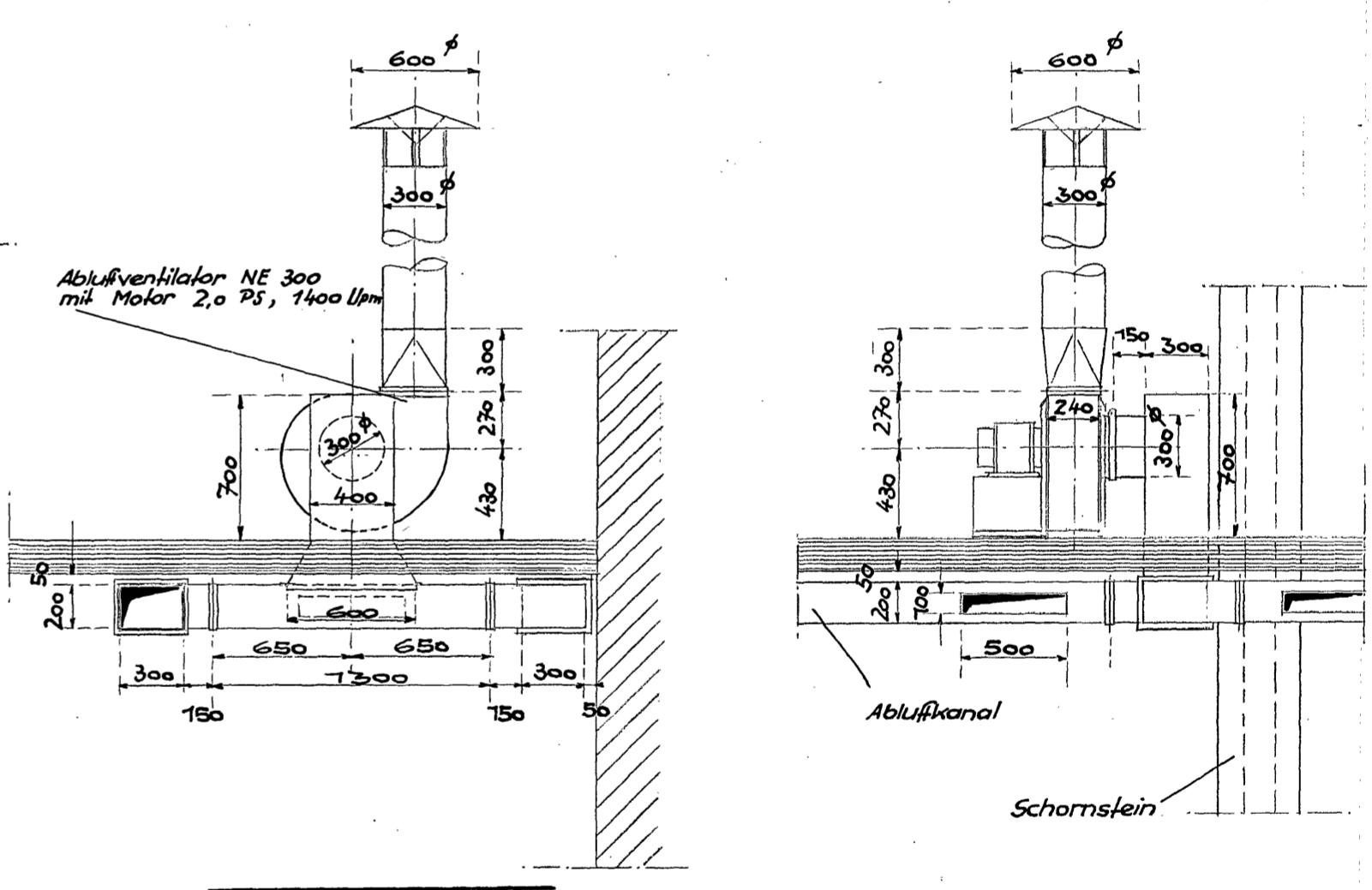
Schnitt E - F
