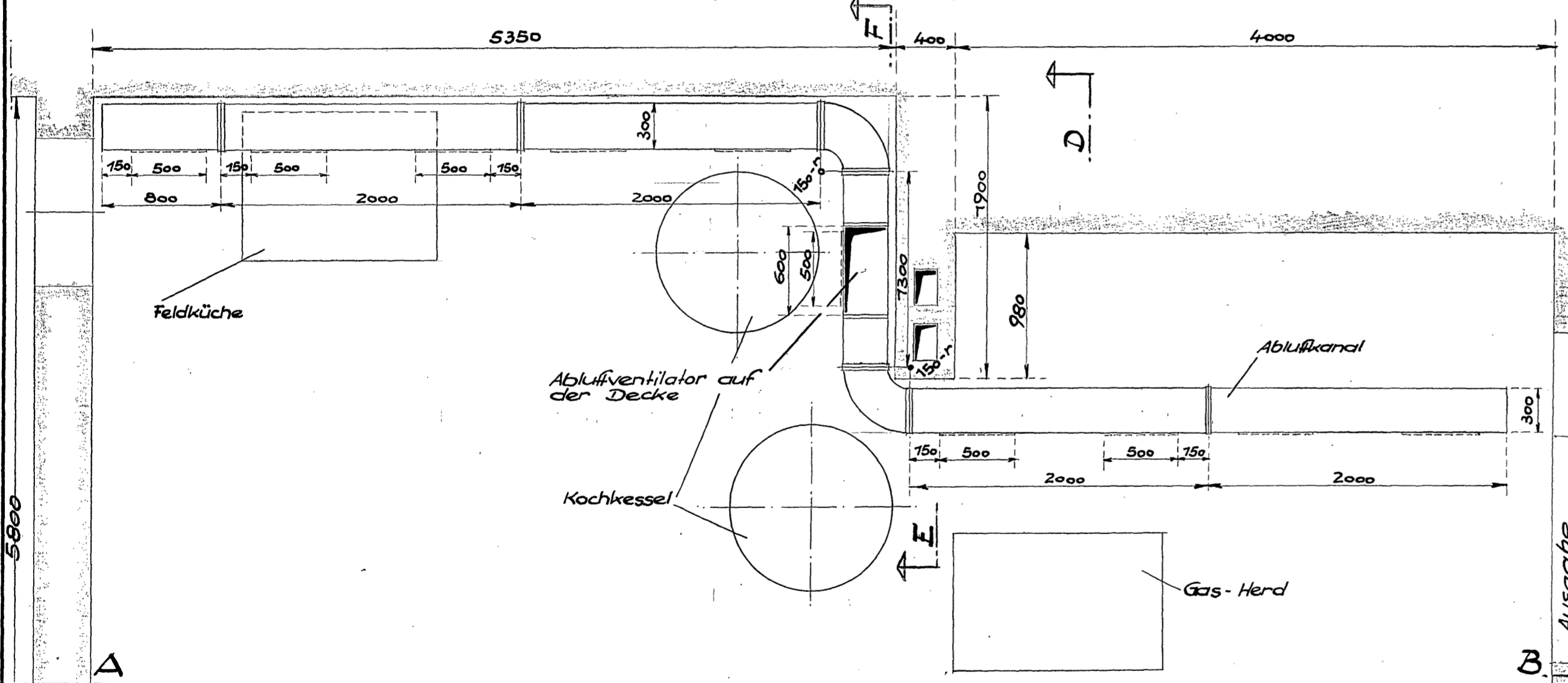
Schnitt A - B
